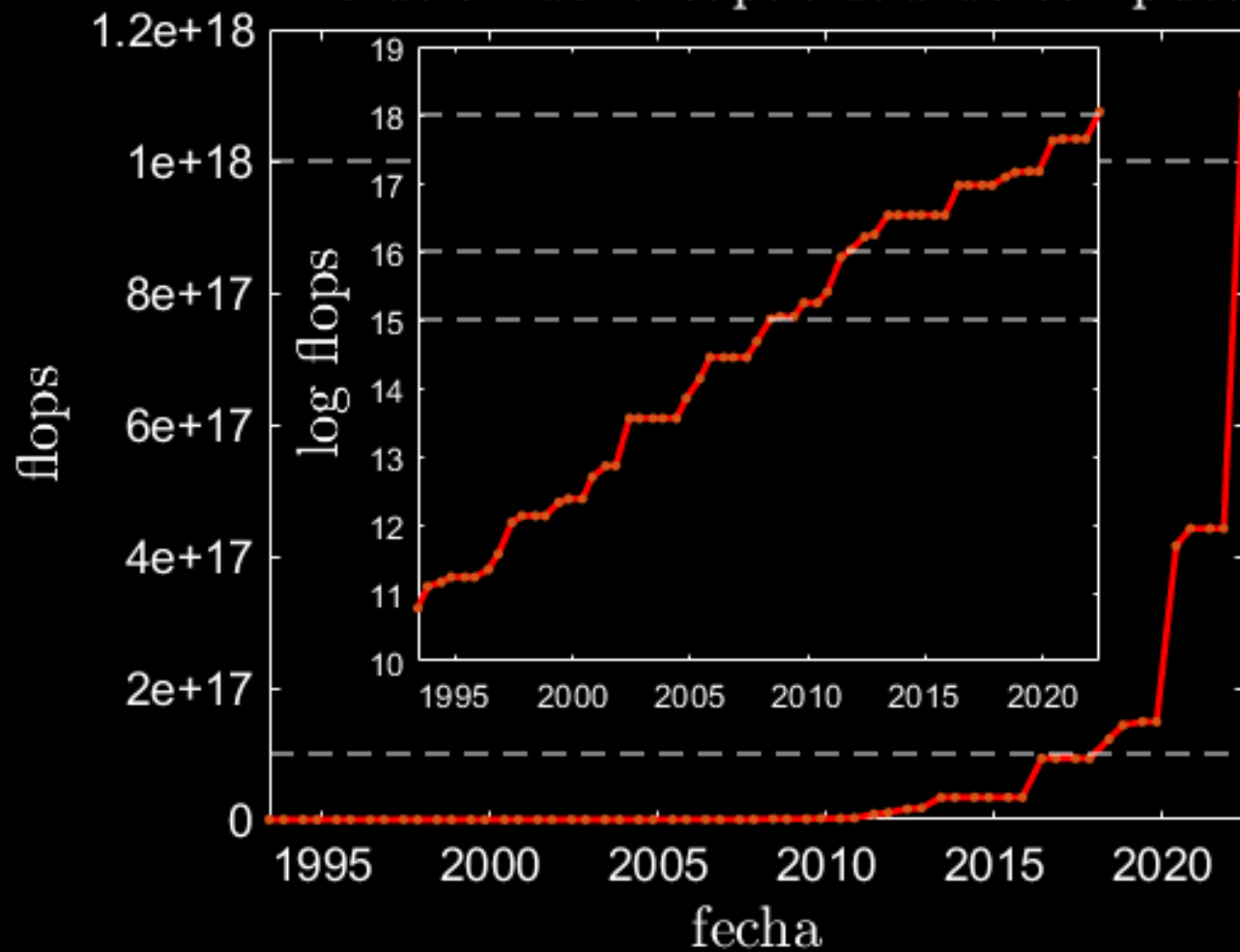
Evolución de la capacidad de cómputo
