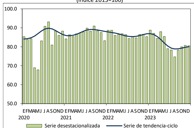
Gráfica 1 SERIE DESESTACIONALIZADA Y DE TENDENCIA-CICLO 2 DE LA PRODUCCIÓN MINEROMETALÚRGICA a diciembre de 2023 (índice 2013=100)
