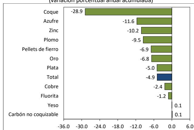
Gráfica 3 VARIACIÓN DE LA PRODUCCIÓN MINEROMETALÚRGICA enero-diciembre p/ de 2023 (variación porcentual anual acumulada)
