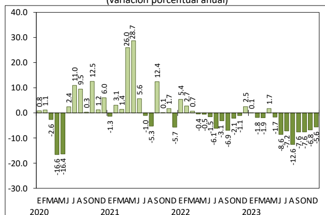
Gráfica 2 VARIACIÓN DE LA PRODUCCIÓN MINEROMETALÚRGICA CIFRAS DESESTACIONALIZADAS a diciembre de 2023 (variación porcentual anual)
