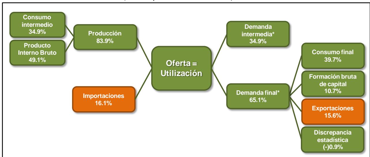
DIAGRAMA OFERTA Y UTILIZACIÓN TOTAL, 2013 (Porcentajes de la oferta/utilización)
