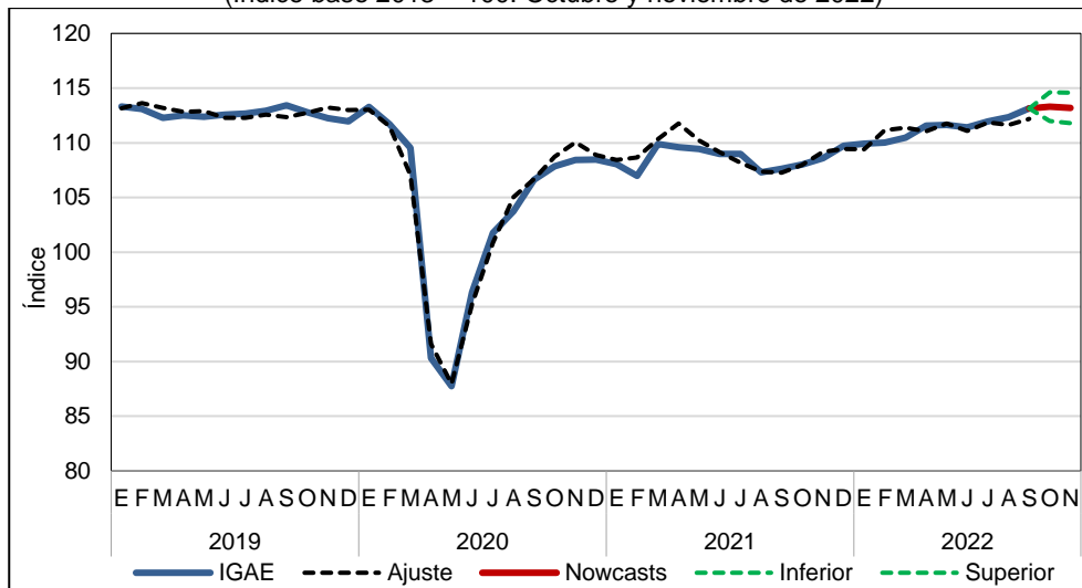
Gráfica 5 IOAE: NOWCAST DEL IGAE MODELOS ESTIMADOS CON SERIES DESESTACIONALIZADAS (Índice base 2013 = 100. Octubre y noviembre de 2022)
