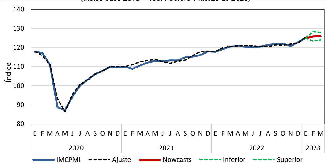
Gráfica 3 IOCP: NOWCAST DEL IMCPMI CIFRAS DESESTACIONALIZADAS (Índice base 2013 = 100. Febrero y marzo de 2023)
