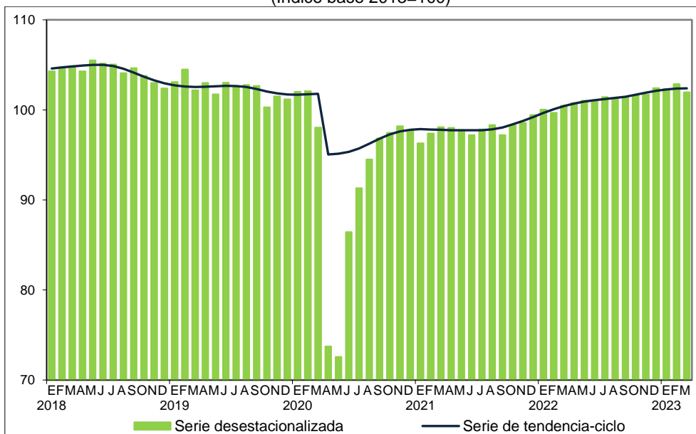
INDICADOR MENSUAL DE LA ACTIVIDAD INDUSTRIAL (Índice base 2013=100)
