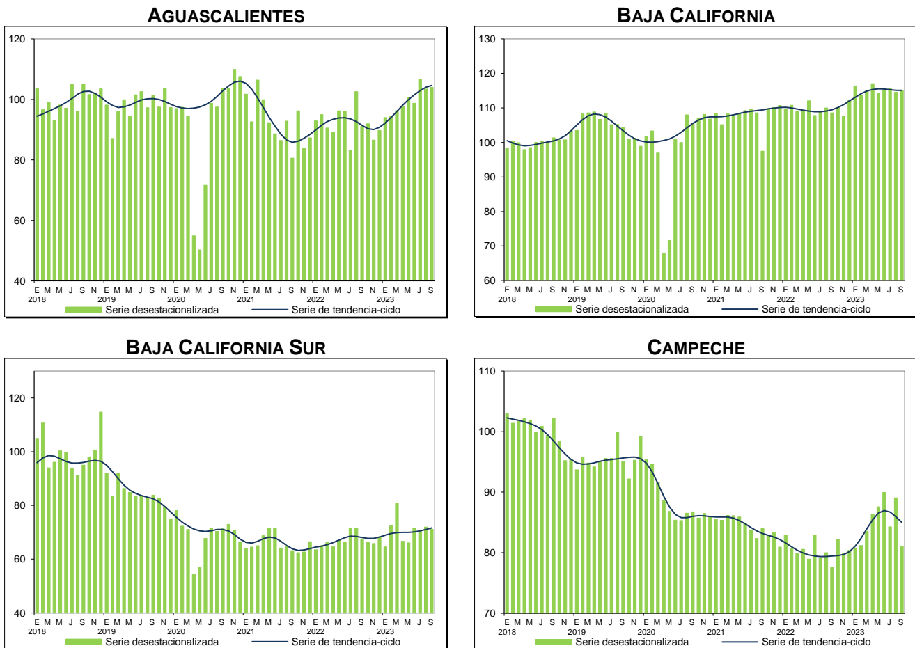
Gráfica 1 SERIE DESESTACIONALIZADA Y DE TENDENCIA-CICLO DE LA ACTIVIDAD INDUSTRIAL POR ENTIDAD FEDERATIVA a septiembre de 2023 (índice 2018=100)
