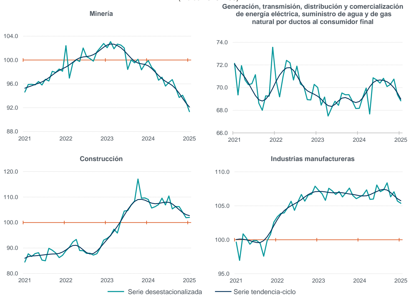
Gráfica 3 Serie desestacionalizada y de tendencia-ciclo de los componentes de la actividad industrial enero de 2021 a enero de 2025 (índice 2018=100)
