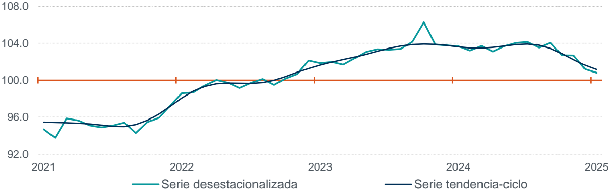
Gráfica 2 Serie desestacionalizada y de tendencia-ciclo de la actividad industrial enero de 2021 a enero de 2025 (índice 2018=100)
