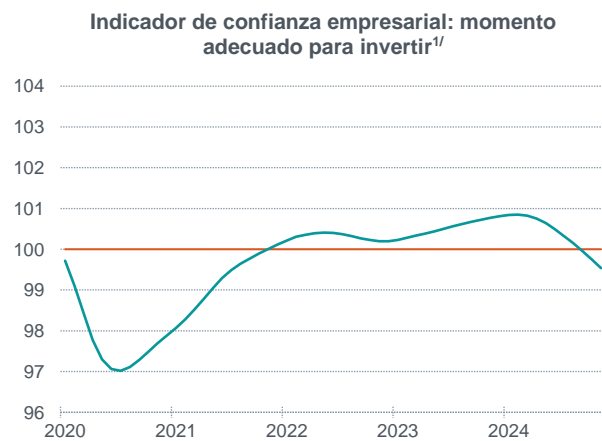
Gráfica 6 Ciclo de los componentes del Indicador Adelantado enero de 2020 a noviembre de 2024 (puntos)
