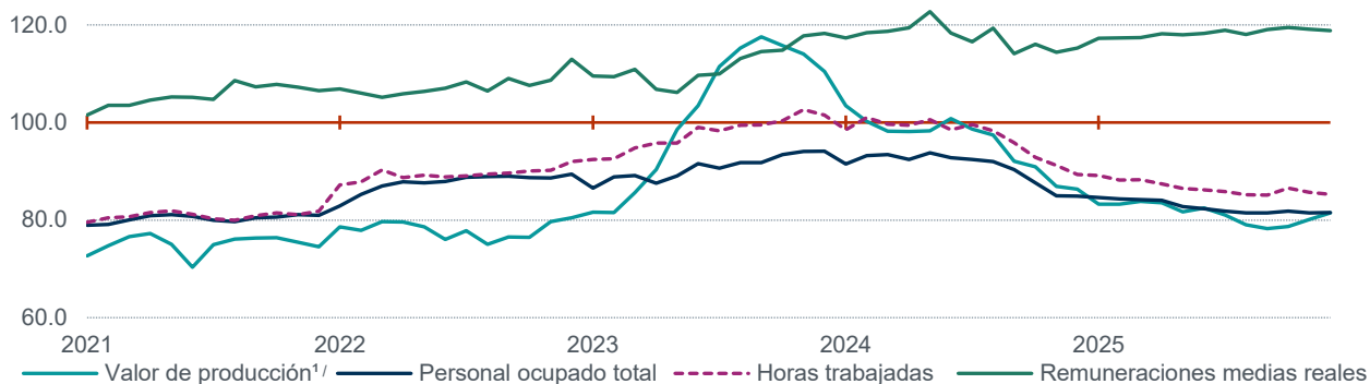
Gráfica 2 Serie desestacionalizada de los indicadores de empresas constructoras enero de 2021-diciembre de 2025 (índice 2018=100)
